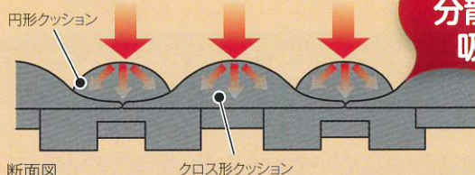
断面図
